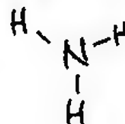
\text{NH}_3 , AMMONIA
